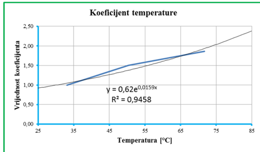
Slika 7-14: Dijagram koeficijenta temperature frakcije 0/11 RA s prikazanom regresijom
