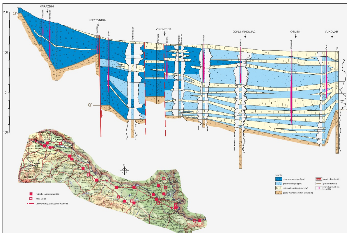
Slika 4.5. Shematski hidrogeološki profil dravskog aluvijalnog vodonosnika (Rudarsko geološko naftni fakultet, 2016.)
