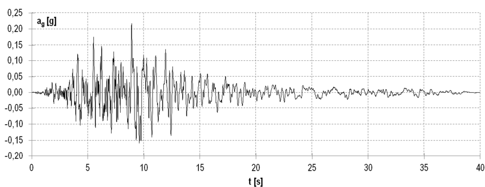
Slika B1.7 Prikaz akceleroograma, spektra energije i idealiziranih spektara ubrzanja i pomaka za zapis potresa Campano Lucano_y.
