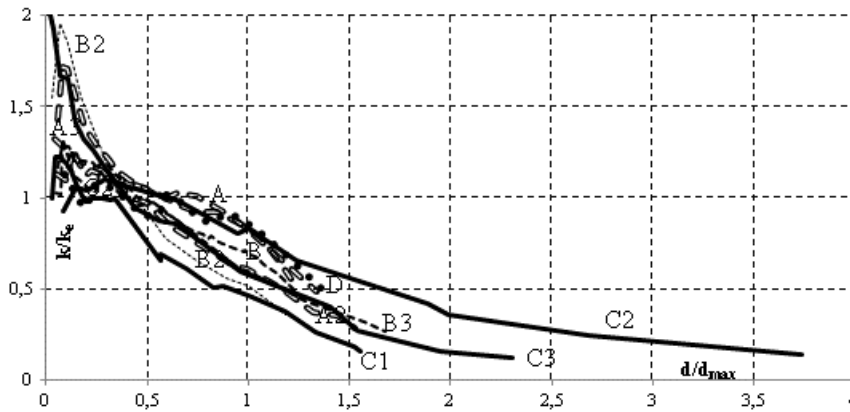
Slika 4.133. Promjena omjera krutosti \frac{K}{K_e} svih uzoraka ovisnosti o omjeru relativnog pomaka \frac{d}{d_{Vax}} (prikaz rezultata pojedinih uzoraka)
