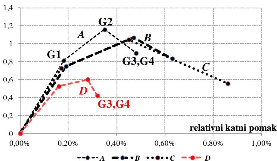
Slika 4.127. Normalizirane krivulje oštećenja uzoraka A,B,C i D
