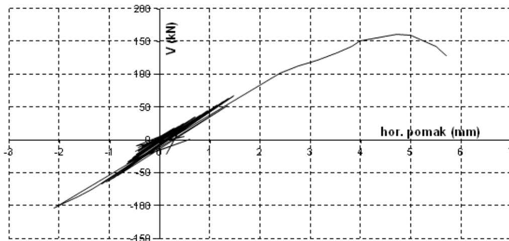
Slika 4.22. Histerezna petlja uzorka A1
