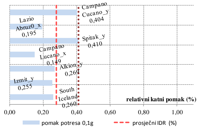
Slika A8. Procijenjeni pomaci dvoetažne građevine gustoće žida d_{wA}=2,46\% za potrese projektnog ubrzanja 0.1g, 0.2g i 0.3g
