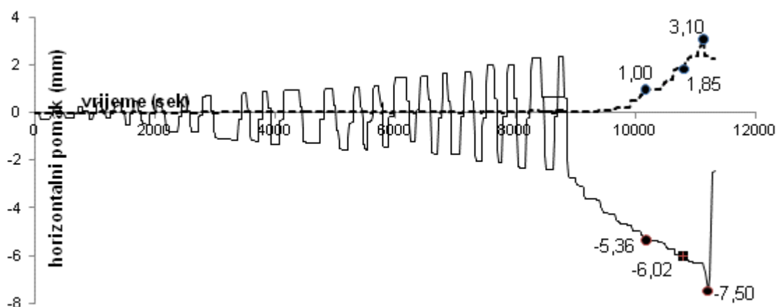
Slika 4.50. Odnos veličine ukupnog mjenjenog horizontalnog i pomaka od smicanja uzorka B1
