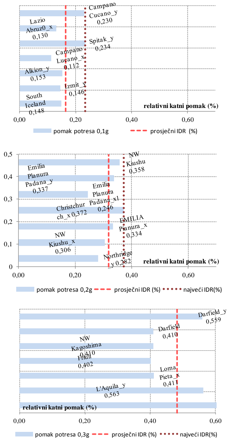
Slika A11. Procijenjeni pomaci dvoetažne građevine gustoće žiđa d_{wA}=5\% za potrese projektnog ubrzanja 0.1g, 0.2g i 0.3g
