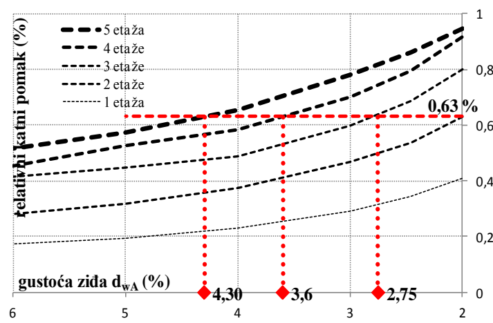
Slika 6.18. Relativni katni pomaci za nivo potresa do 0,2g
