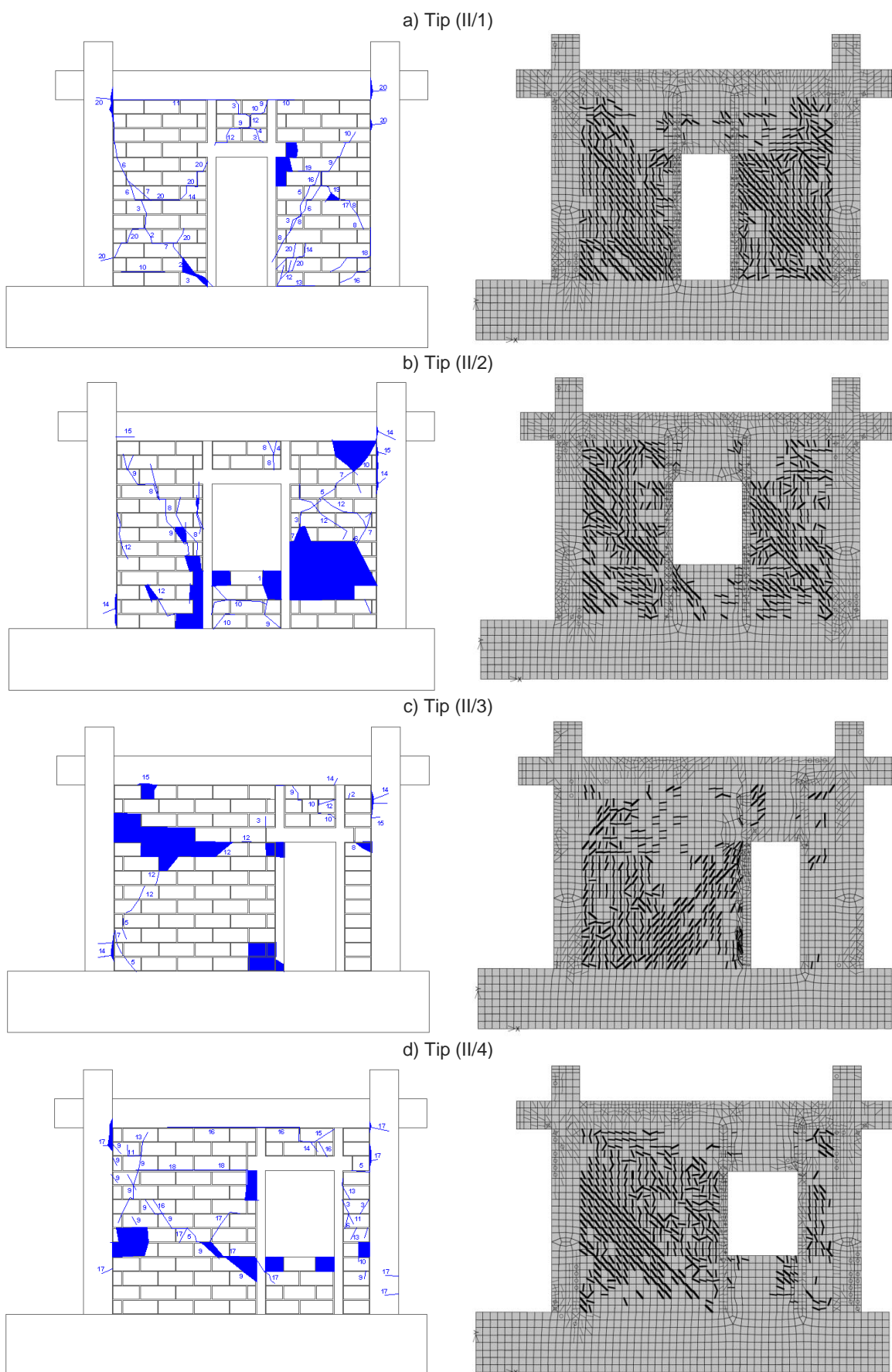
Slika 5.19. Usporedba eksperimentalnih (lijevo) i numeričkih rezultata (desno) ispitnih uzoraka: a) Tip (II/1), b) Tip (II/2) , c) Tip (II/3) i d) Tip (II/4)
