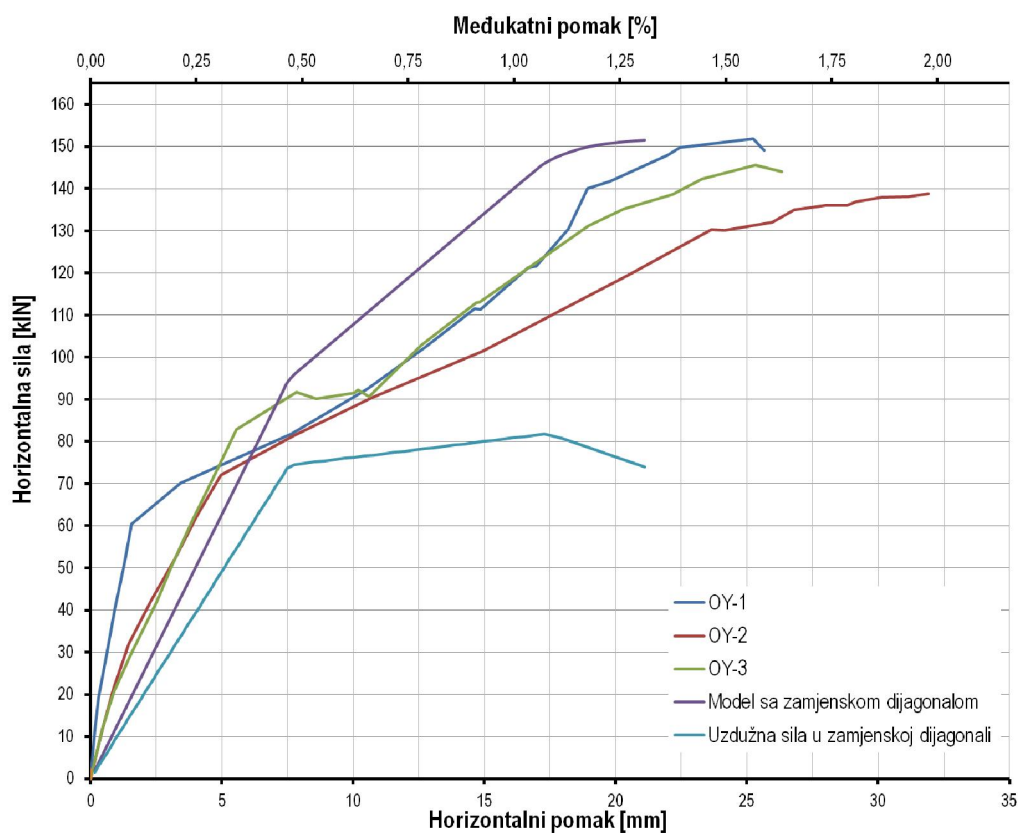
Slika 5.9 – Dijagram horizontalna sila - horizontalni pomak za okvire OY-i i model sa zamjeskom dijagonalom
