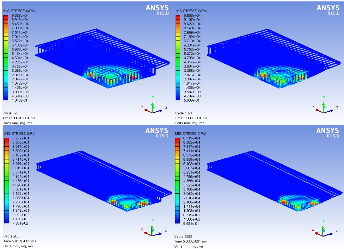
Slika 9.12 – Mises naprezanje armature rasponskog sklopa u t=0,5 ms
