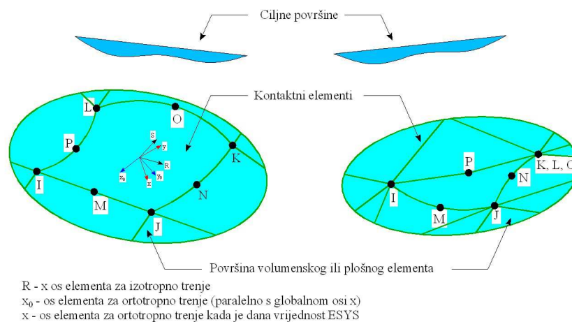
Slika 6.14 – CONTA174
