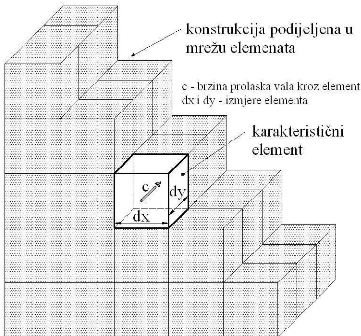
Slika 5.1 – Karakteristični konačni element
