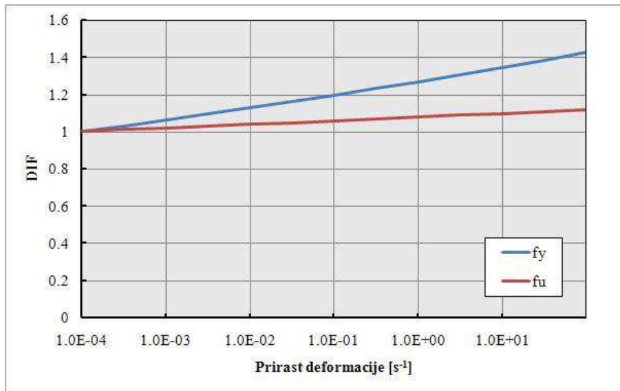
Slika 7.14 – DIF za armaturni čelik
