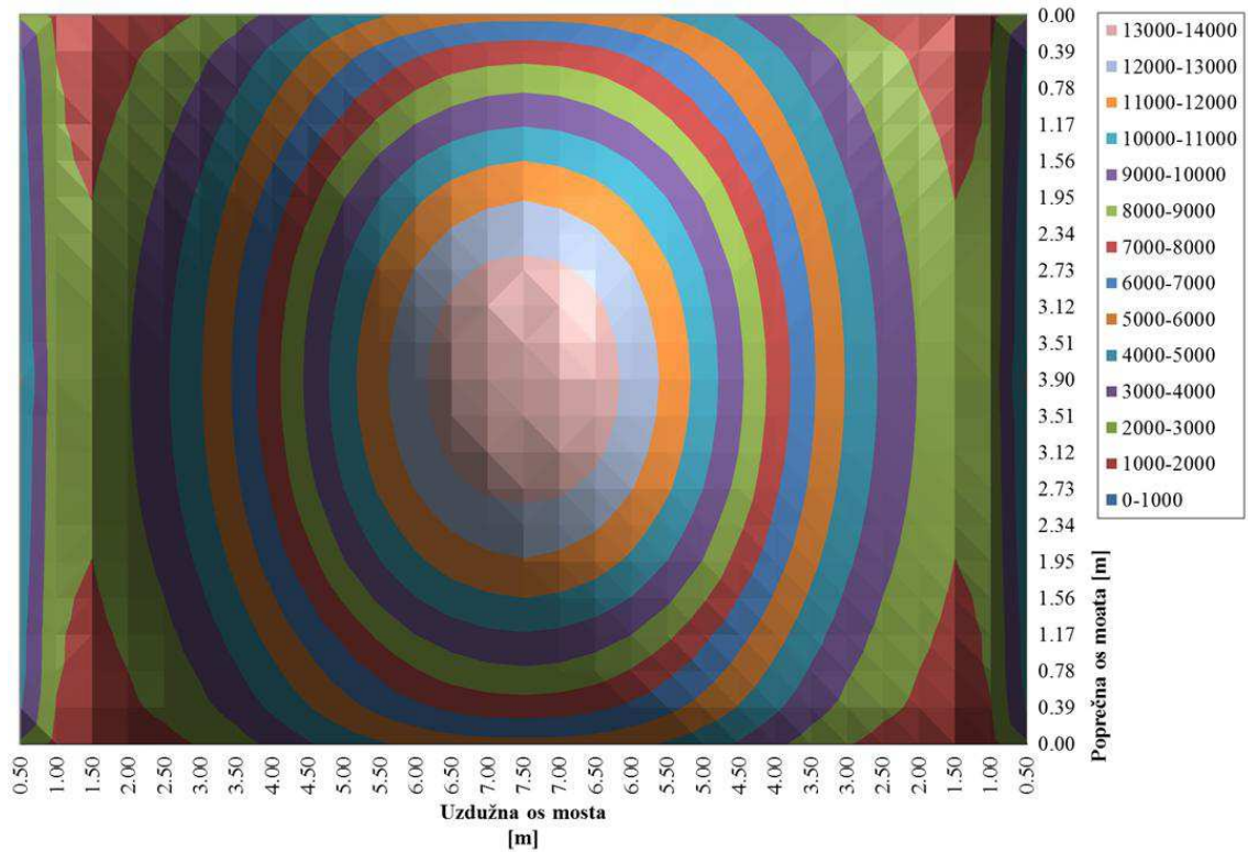
Slika 6.25 – Anvelopa maksimalnih tlakova na rasponski sklop mosta Tip 1
