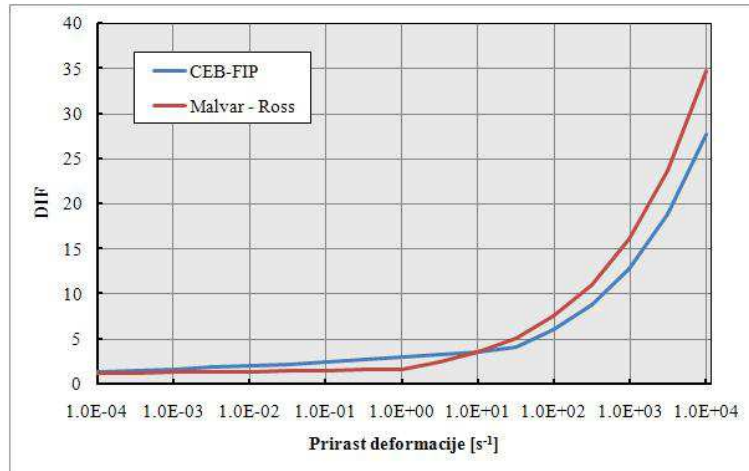
Slika 7.11 – DIF za vlačnu čvrstoću betona
