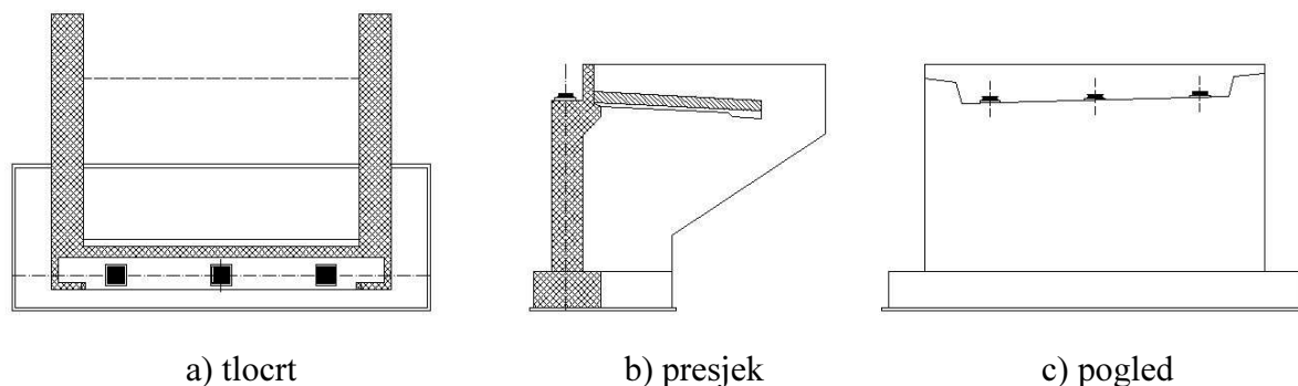
Slika 6.4 – Masivni upornjak
