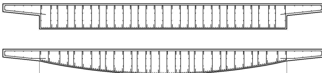
Slika 6.3 – Raspored armature pločastog sklopa
