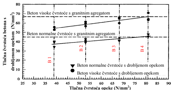
Slika 2. 5: Ovisnost tlačne čvrstoće betona s drobljenom opekama i tlačne čvrstoće opeke, [16]
