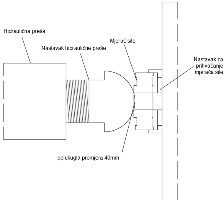
Slika 33. Prikaz spoja hidraulične preše, mjerča sile i modela konstrukcije.
