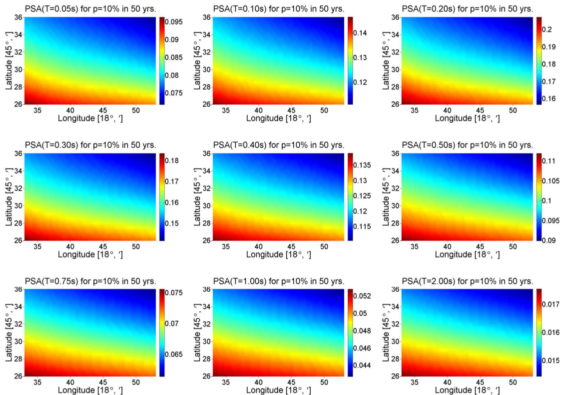
Slika 3.9 Vrijednosti niza spektralnih amplituda za duboko aluvijalno tlo, dobivene probalističkim proračunom potresne opasnosti za promatrano područje, upotrebom atenuacijskih jednadžbi za spektralne amplitude Sabetta i Pugliese (1996.), za vjerojatnost 10 % u 50 godina (povratno razdoblje od 475 godina)
