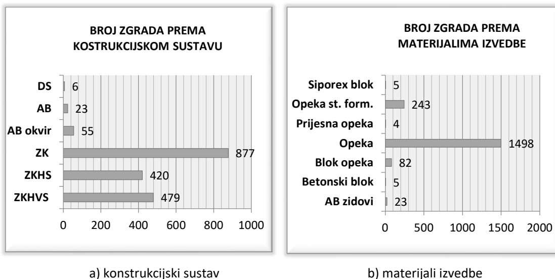
Slika 4.18 Brojnost zgrada prema konstrukcijskom sustavu i materijalima izvedbe u modelu izloženosti grada Osijeka
