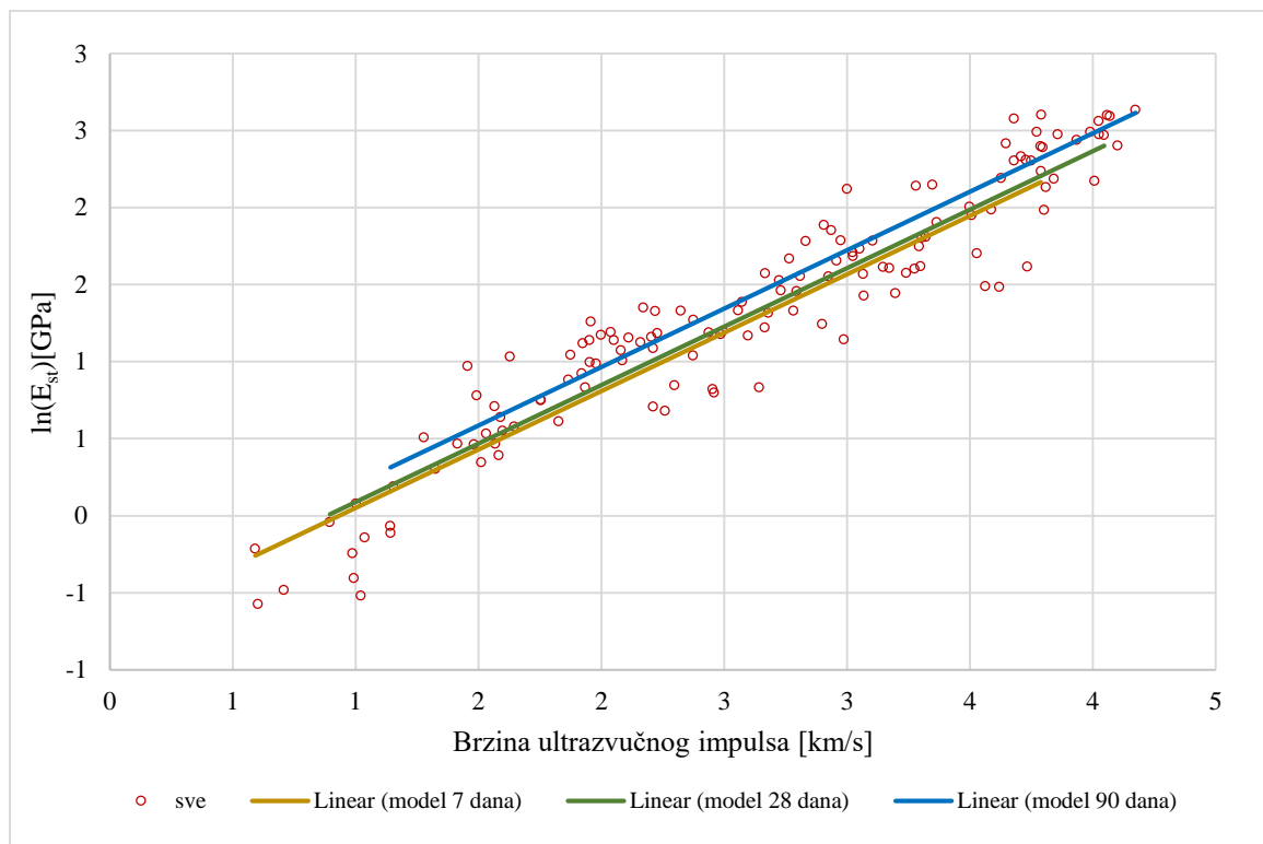
Slika 5.9. Korelacija brzine ultrazvučnog impulsa i statičkoga modula elastičnosti transformiranog prirodnim logaritmom
