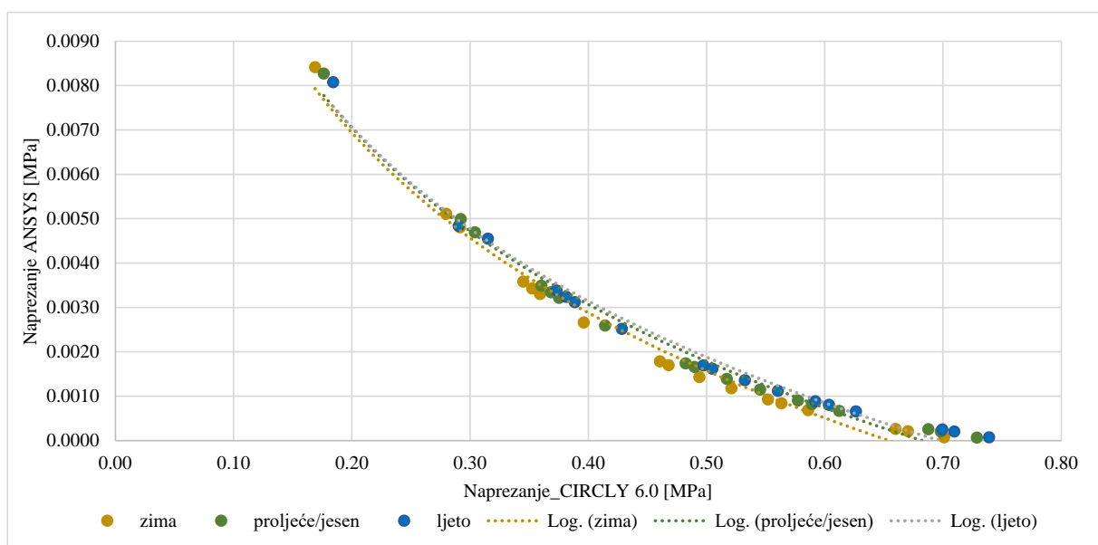
Slika 7.15. Veza između naprezanja u CNS-u izračunatih pomoću dva računalna programa
