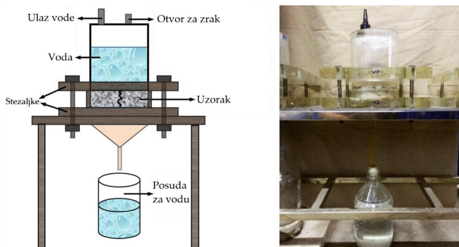
Slika 2.12. Ispitivanje vodopropusnosti [36]
