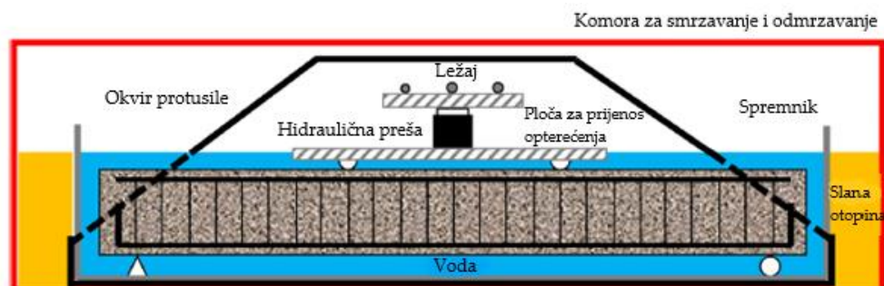
Slika 5.4. Shematski prikaz prethodnog opterećenja greda uz istodobno smrzavanje/odmrzavanje
