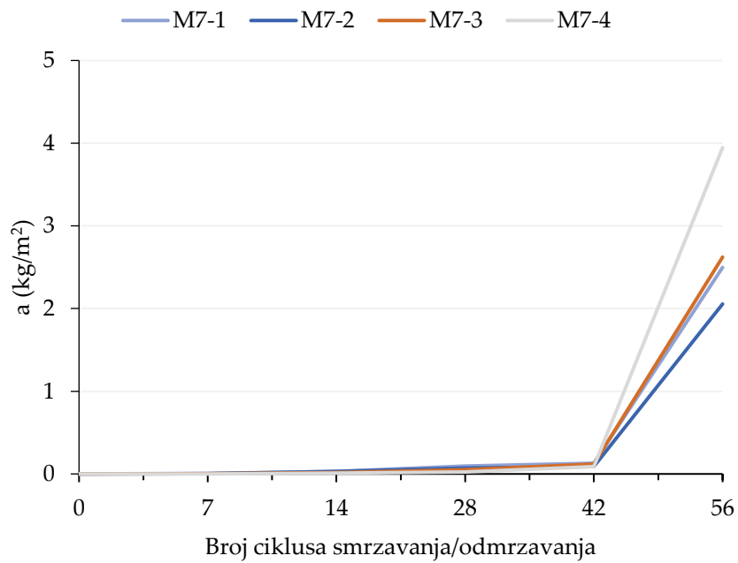
Prilog 30. Pojedinačni rezultati ispitivanja količine oljuštenog materijala po jedinici površine uslijed ciklusa smrzavanja i odmrzavanja bez soli mješavine M7
