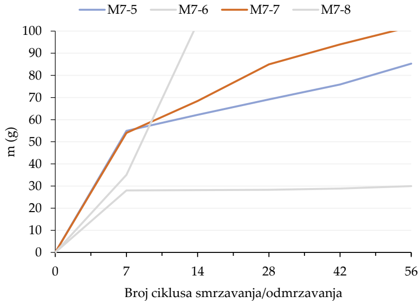
Prilog 15. Pojedinačni rezultati ispitivanja gubitaka mase ljuštenjem uslijed ciklusa smrzavanja i odmrzavanja sa soli mješavine M7
