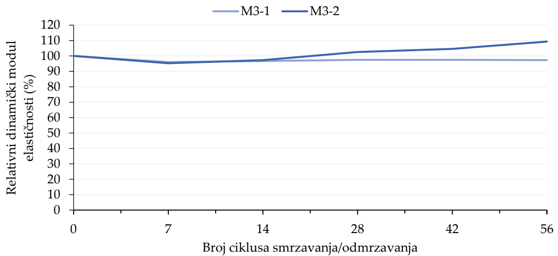
Prilog 38. Pojedinačni rezultati ispitivanja unutarnjih oštećenja uslijed ciklusa smrzavanja i odmrzavanja bez soli mješavine M3
