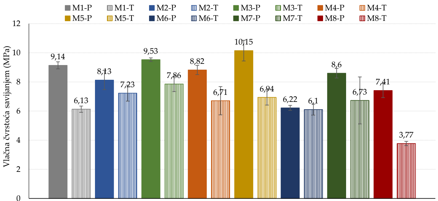
Slika 6.47. Rezultati ispitivanja vlačne čvrstoće savijanjem betona svih mješavina nakon i prije smrzavanja
