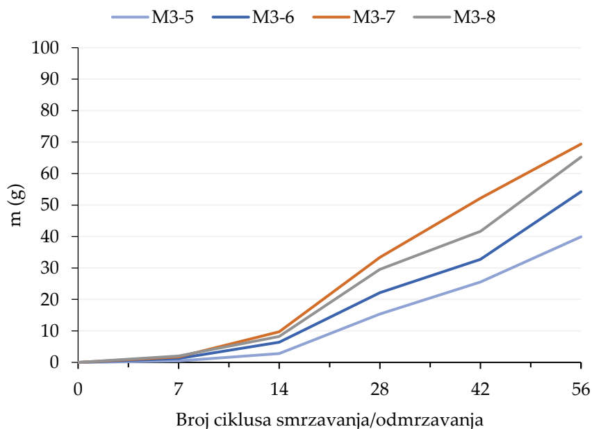
Prilog 7. Pojedinačni rezultati ispitivanja gubitaka mase ljuštenjem uslijed ciklusa smrzavanja i odmrzavanja sa soli mješavine M3
