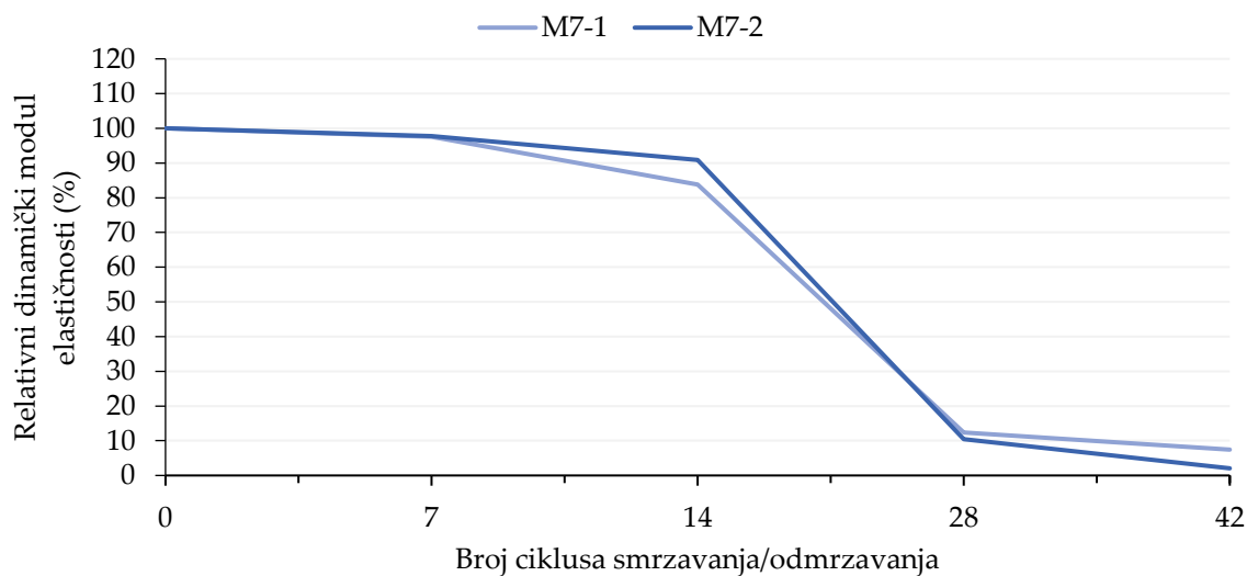
Prilog 46. Pojedinačni rezultati ispitivanja unutarnjih oštećenja uslijed ciklusa smrzavanja i odmrzavanja bez soli mješavine M7
