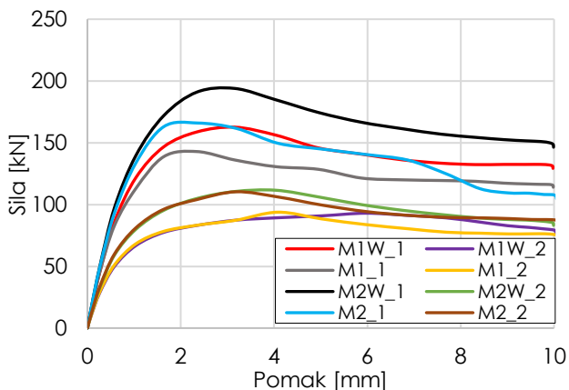
Slika 4. Odnos sile i pomaka
