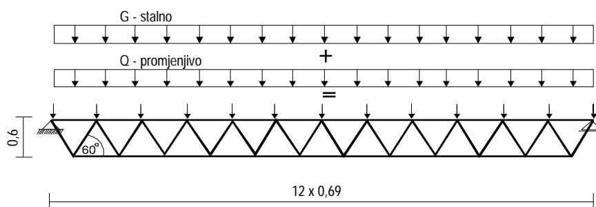
Slika 1 – Rešetkasta konstrukcija i opterećenje
