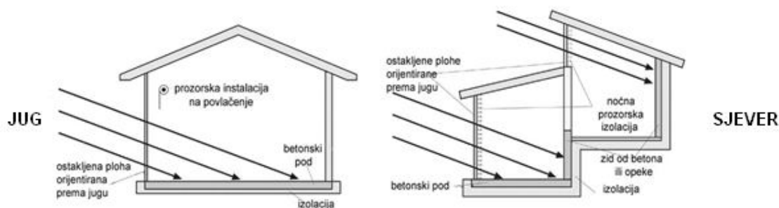
Slika 4 - Direktni zahvat Sunčevog zračenja
