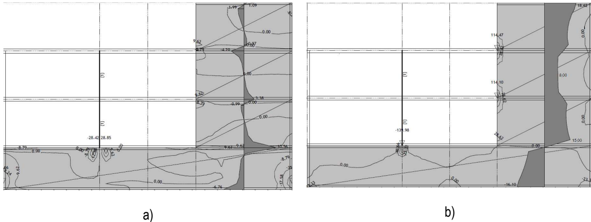
Slika 10 – Presjek 4-4 poprečna sila V_{z,x} (a) i poprečna sila V_{z,y} (b)
