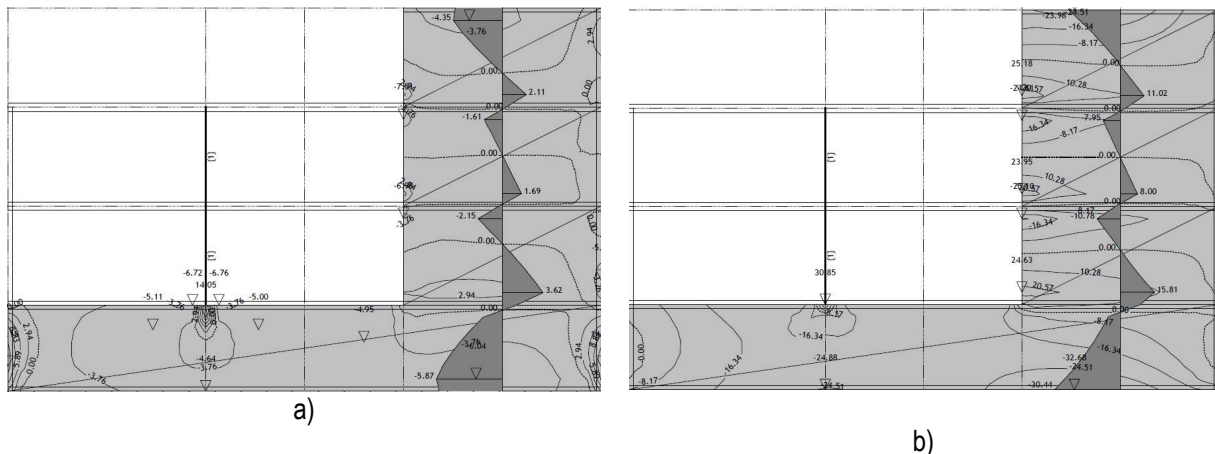
Slika 9 – Presjek 4-4 moment savijanja M x (a) i moment savijanja M y (b)
