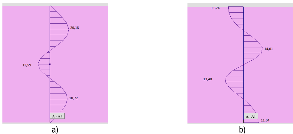
Slika 6 – Moment savijanja M_y u presjeku 1-1 (a) i poprečna sila V_{z,y} (b)
