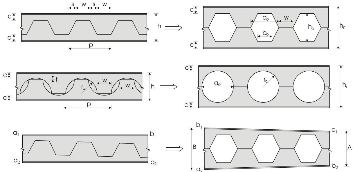
Slika 1 – Sačasti nosači
