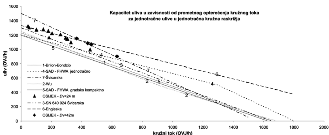
Slika 6 Usporedba kapaciteta uliva za jednostručne ulive u jednostručna kružna raskrižja Figure 6 Comparison of the capacity for the single-line approach and single-line roundabout
