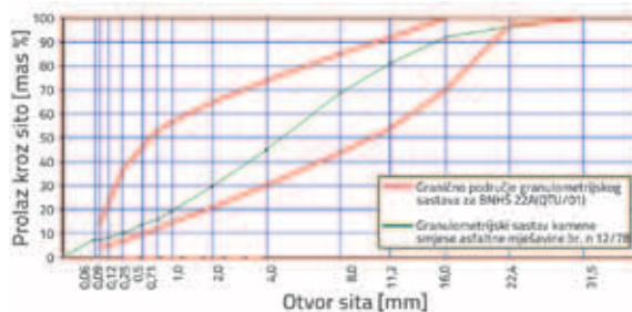
Slika 4. Granulometrijski sastav asfaltne mješavine s 15% recikliranog asfalta [5]
