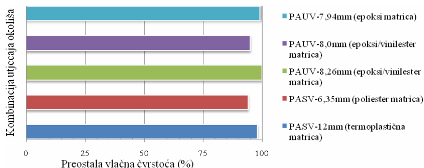
Slika 4. Vrijednosti preostale vlačne čvrstoće pri kombinaciji djelovanja okoliša (tablica 4.) za šipke od PAV-a [10]
