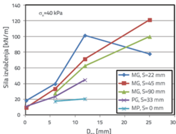
Slika 17. Utjecaj promjera zrna tla na silu izvlačenja kod metalnih i polimerne mreže te metalne ploče [3]
