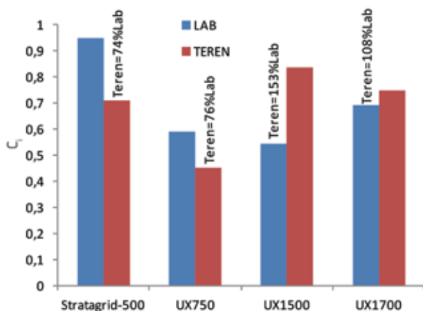
Slika 21. Usporedba koeficijentata interakcije kod modelskog i terenskog pokusa izvlačenja [58]
