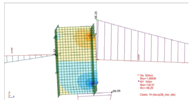
Slika 7. Primjer prikaza rezultata proračuna primjenom predloženog načina modeliranja
