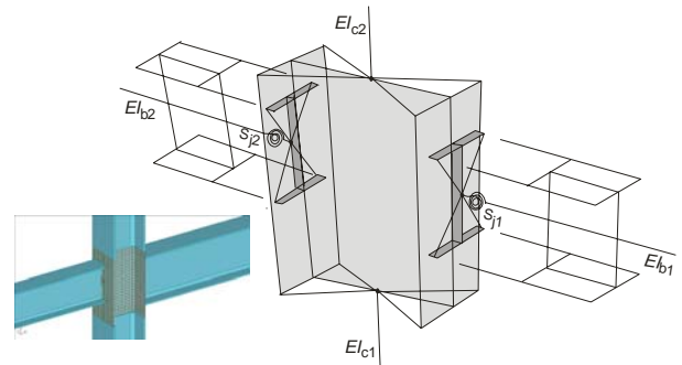
Slika 6. Modeliranje metodom konačnih elemenata priključka i okvirne konstrukcije
