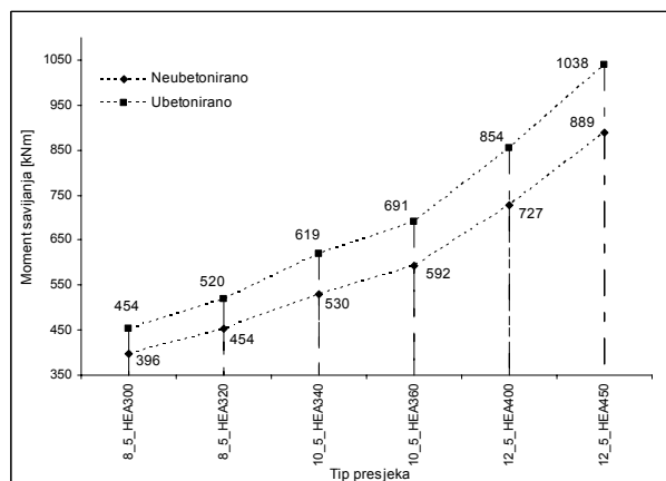
Slika 15. Otpornost spregnutih nosača s HEA presjekom, razmak 5 m
