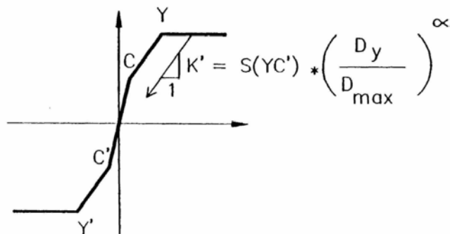
opadajuća krutost u Takedinoj histerezi
