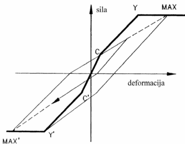
Takeda histereza za sila-deformacija
