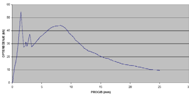
Odnos opterećenje – progib
