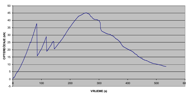
Odnos opterećenje – vrijeme
