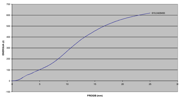
Odnos energija – progib
