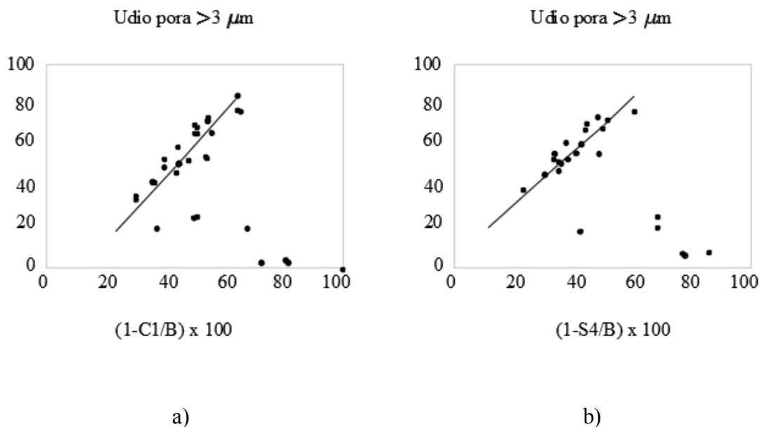
Slika 3.30 Povezanost parametara upijanja vode sa udjelom pora većih od 3 \mu\text{m} : a) povezanost udjela pora većih od 3 \mu\text{m} (P3) s (1-C1/B)*100 , b) povezanost udjela pora većih od 3 \mu\text{m} (P3) s (1-S4/B)*100 [97,127]
