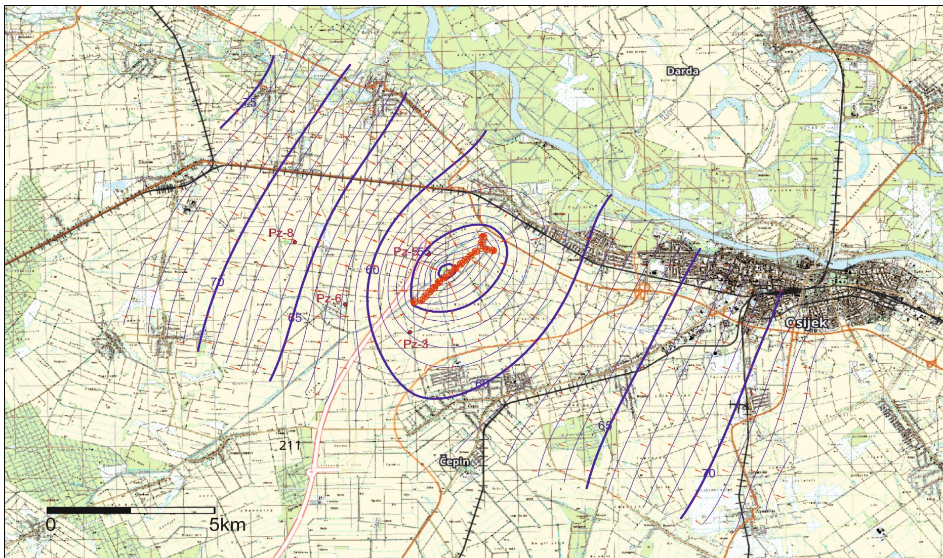
Slika 6.41. Konturna karta piezometarskih razina modeliranog hipotetskog strujanja u vodonosniku za slučaj višegodišnjeg (simulirano 5 godina) ekstremno sušnog razdoblja (godišnja oborina ne prelazi 314 mm) uz povećanje crpnih količina za 15%.
