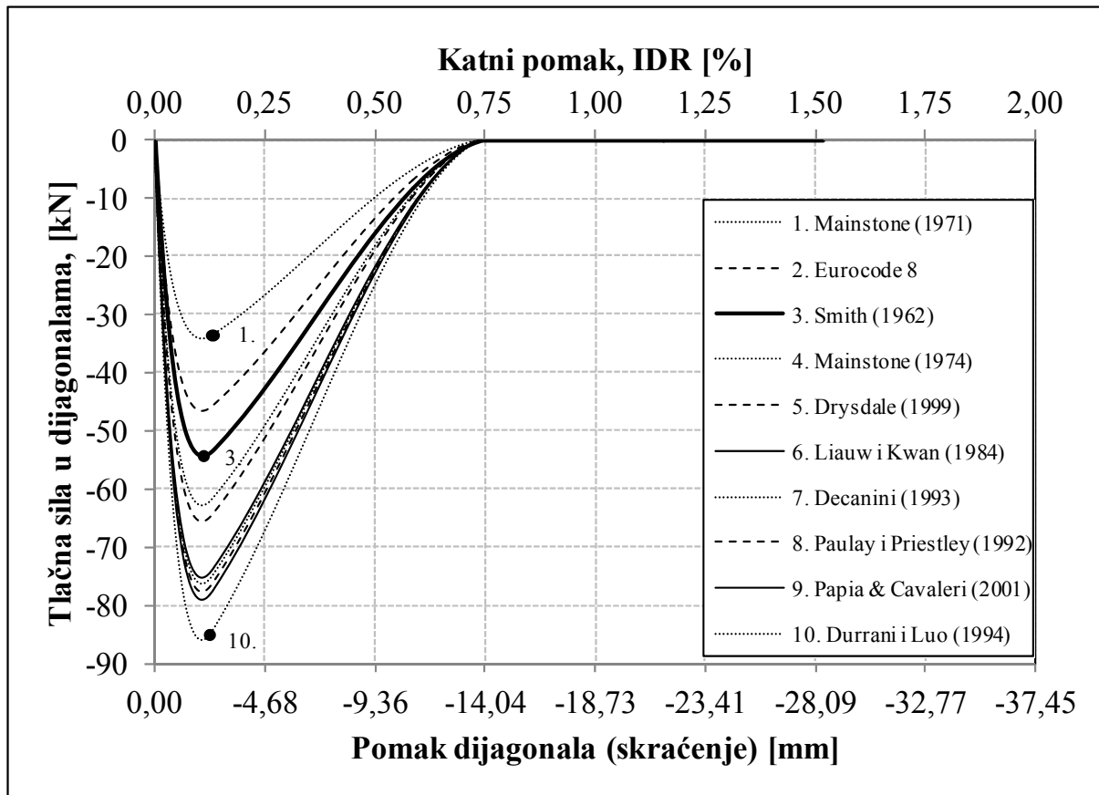
Slika 8.7 Utjecaj širine tlačne dijagonale na silu u tlačnoj dijagonali
