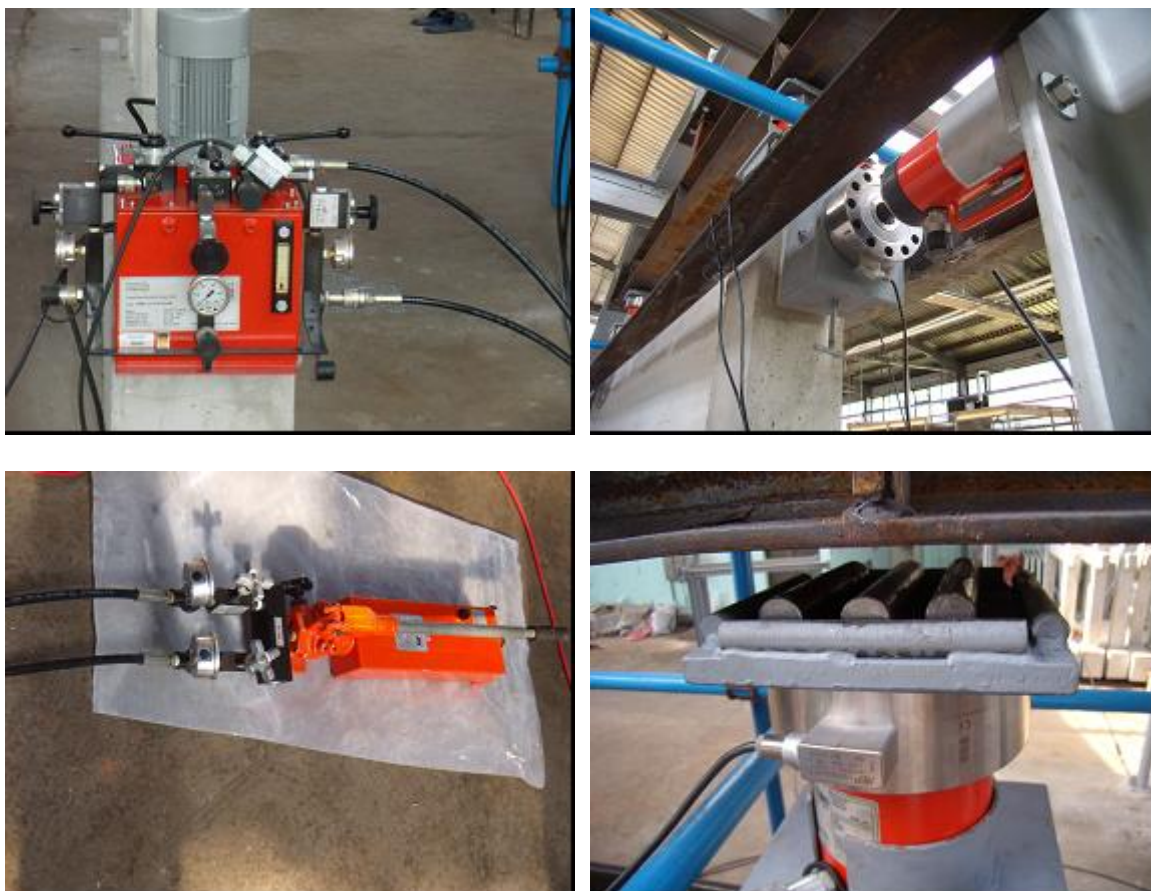
Slika 4.13 Prikaz instrumenata za unos horizontalne i vertikalne sile
