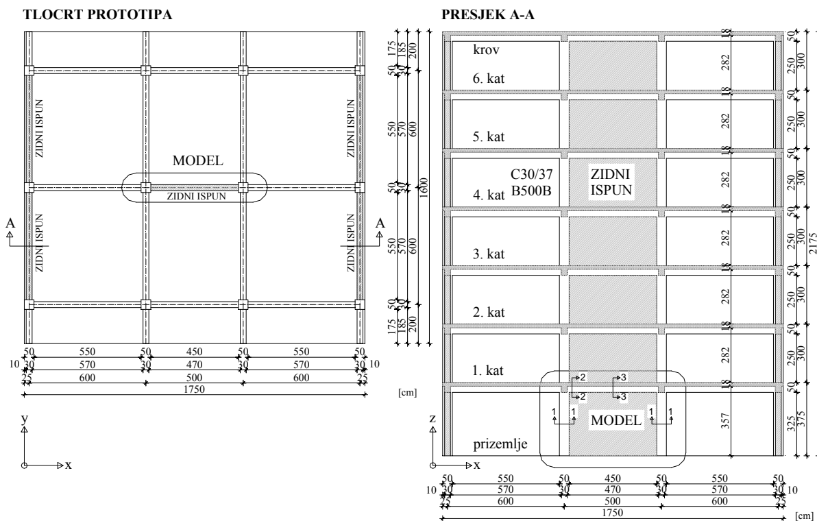
Slika 2.1 Model prototipa
