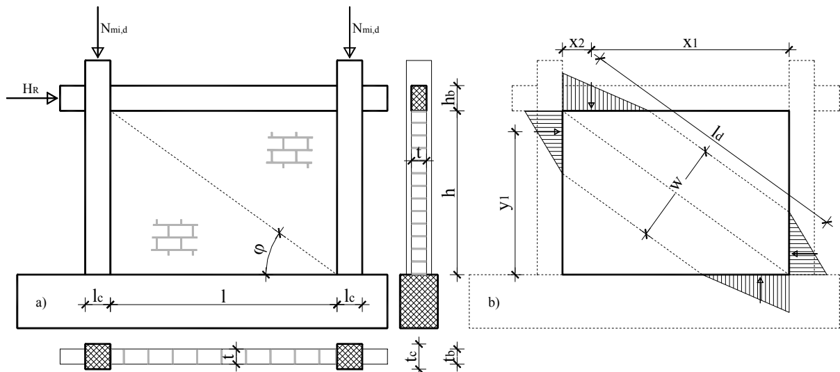
Slika 5.3 a) Skica armirano-betonskog okvira ispunjenog zidnim ispunom, b) Idealizirana napreznja u uglovima tlačne dijagonale
