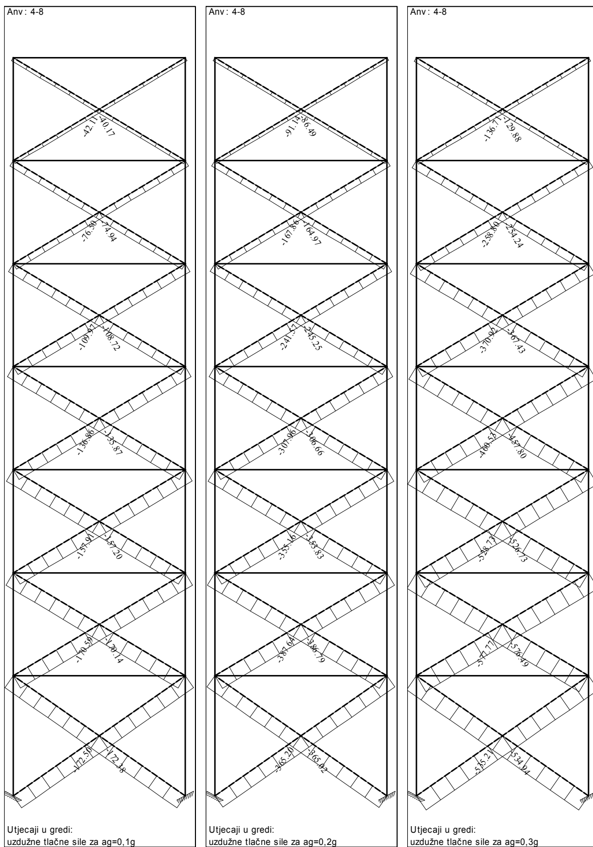
Slika 9.21 Prikaz uzdužnih tlačnih sile u zamjenskim dijagonalama – 7. katova
