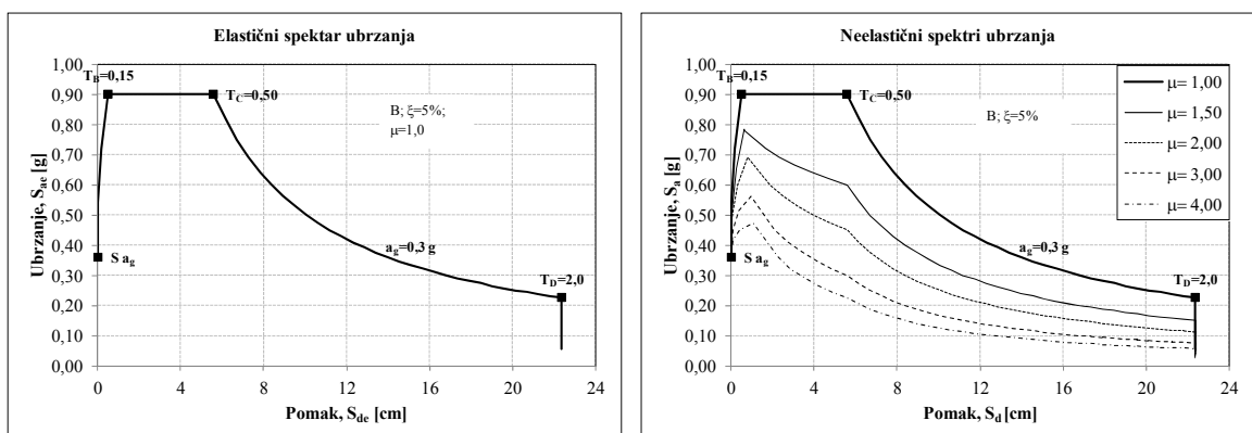
Slika 9.44 Spektri zahtjeva u obliku AD - a_g=0,3g
