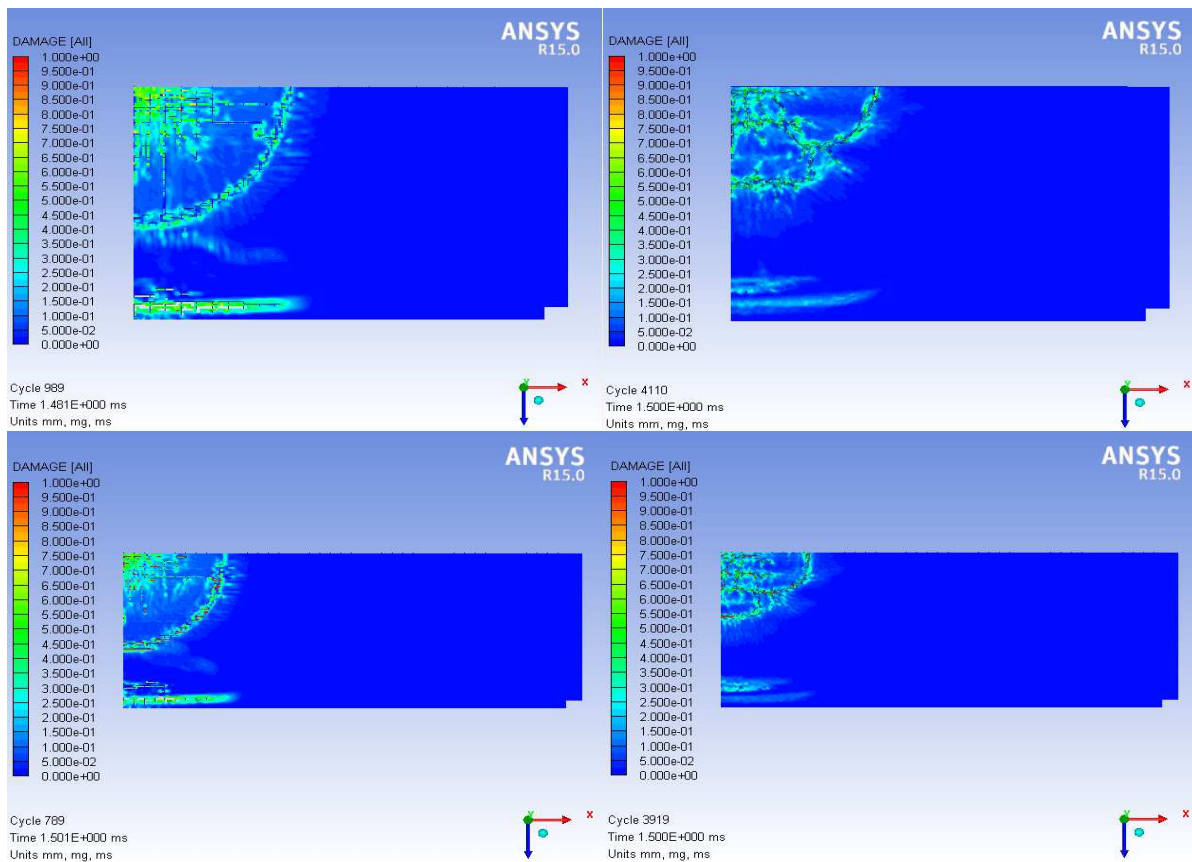
Slika 9.19 – Oštećenje rasponske konstrukcije u t=1,5 ms - gornja ploha
