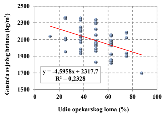
Slika P.1. 24: Korelacija između udjela opekarskog loma i gustoće svježeg betona
