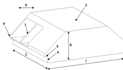
Oznake: 1 rebro 2 dužina bloka 3 gornja ploha bloka 4 širina zuba 5 visina zuba 8 ukupna visina bloka 6 dubina zuba 7 ukupna dužina bloka 9 smjer nosača
