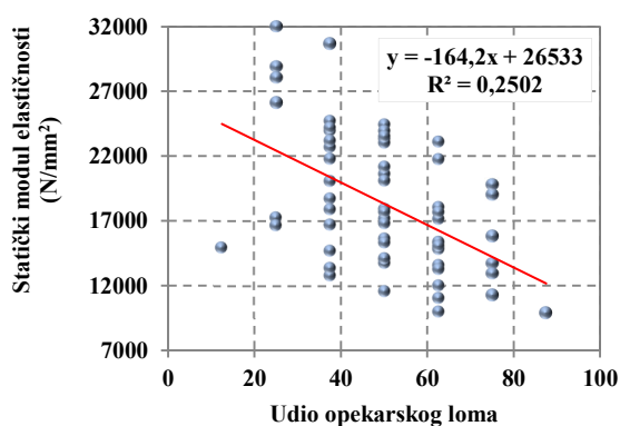
Slika P.1. 4: Korelacija između udjela opearskog loma i statičkog modula elastičnosti
