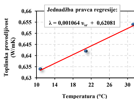
Slika 6. 18: Toplinska provodljivost uzorka betona
