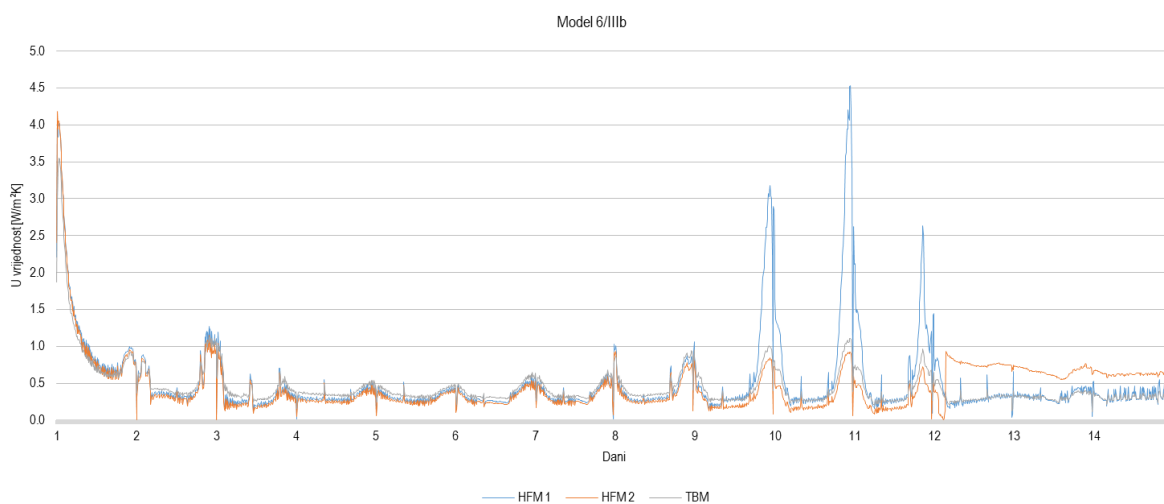
Slika 5.32 Prikaz dobivenih U vrijednosti HFM i temperaturnom metodom tijekom sezone grijanja, model 6/IIb
