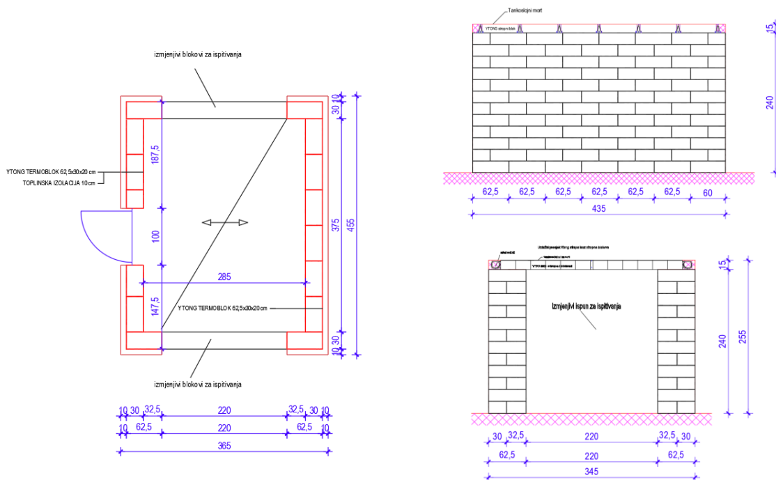
Slika 4.1 Geometrija komore
