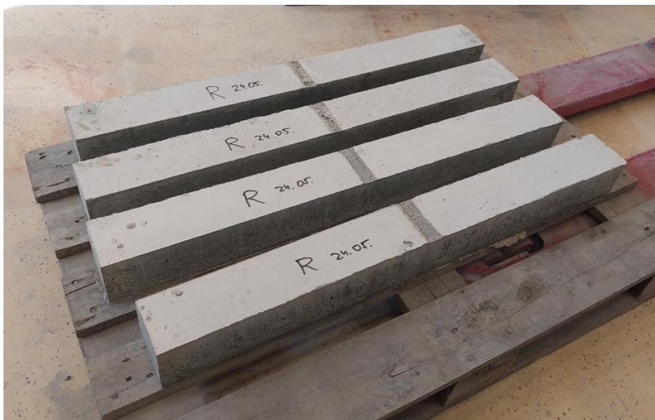
Slika 7.16. Raskalupljene grede referentne mješavine
