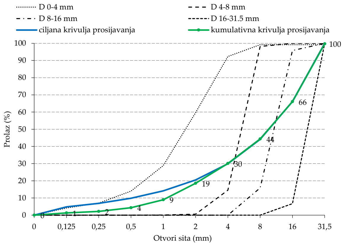
Slika 6.2. Krivulje prosijavanja frakcija, ciljane i stvarna kumulativna krivulja agregata
