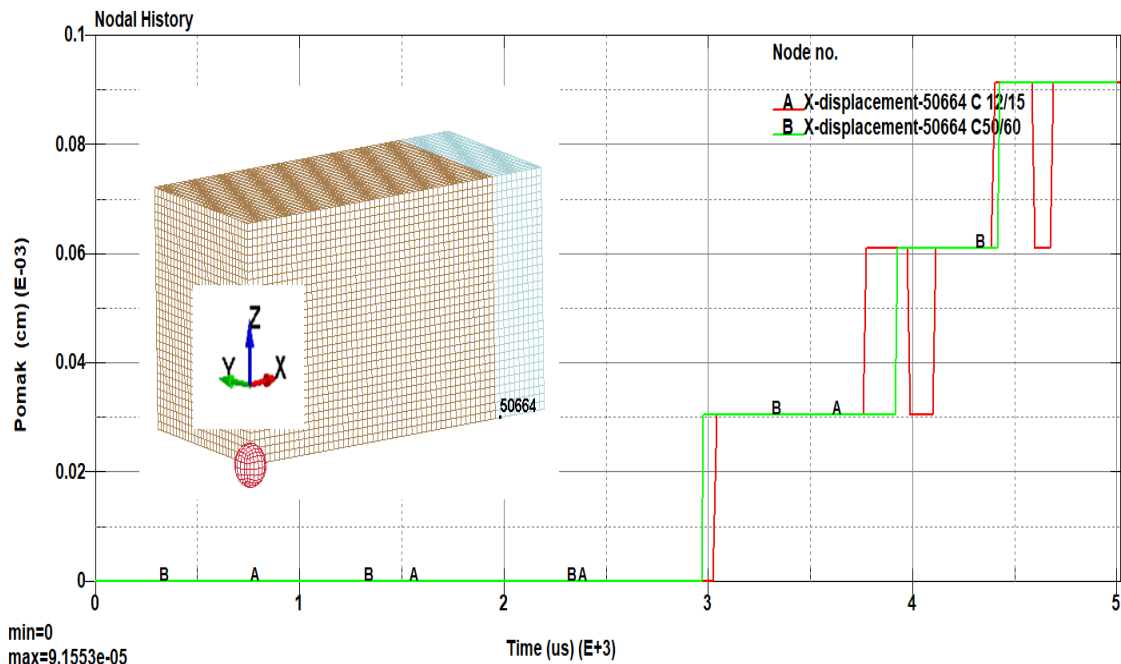
Slika 6.86 Dijagrami horizontalnog pomaka čvorova
