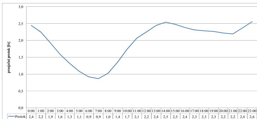
Slika 16 - Dnevni hidrogram
