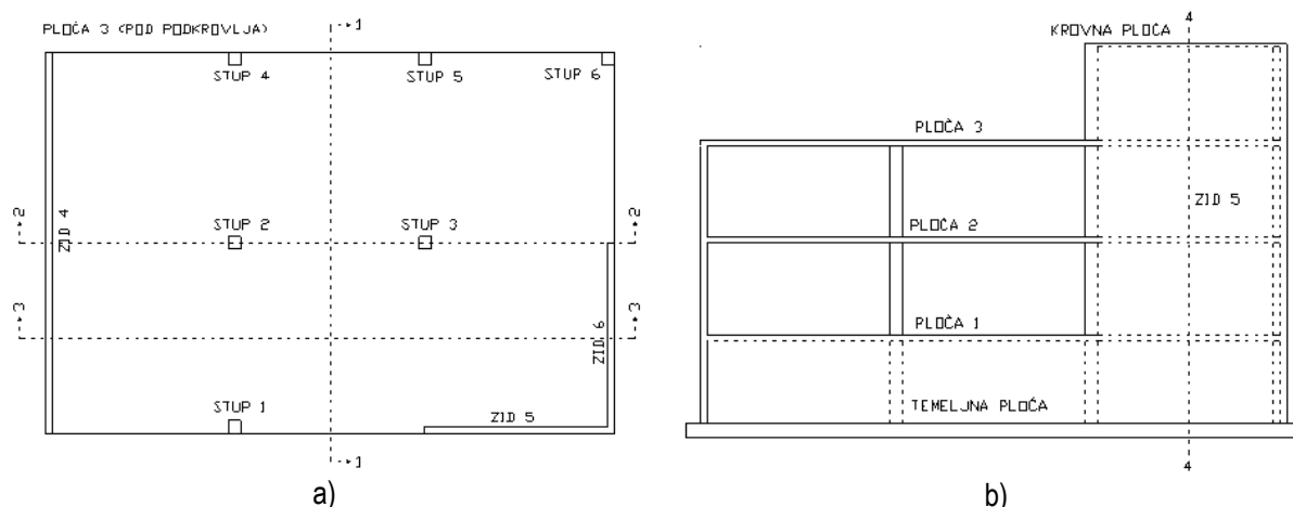
Slika 5 – Mjerodavni presjeci : a) Tlocrt prizemlja i prvog kata, b) Poprečni presjek građevine
