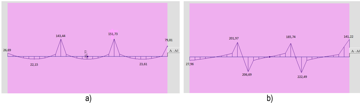
Slika 7 – Presjek 2-2 moment savijanja M_x (a) i poprečna sila V_{z,x} (b)
