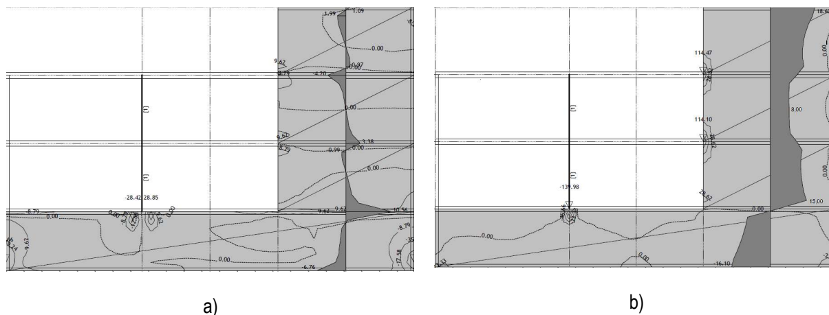
Slika 10 – Presjek 4-4 poprečna sila V_{z,x} (a) i poprečna sila V_{z,y} (b)
