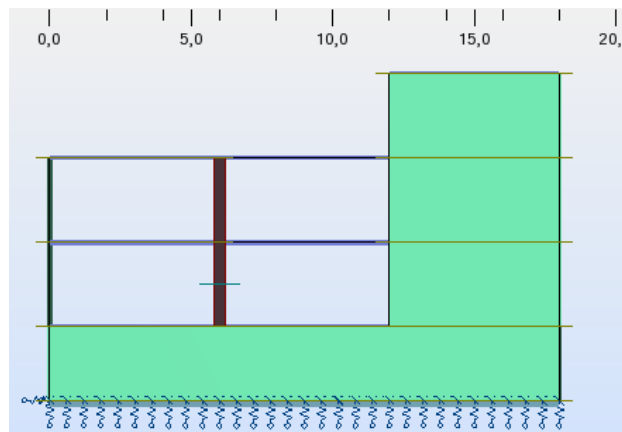
Slika 3 – Modeliranje oslonca temeljne ploče
