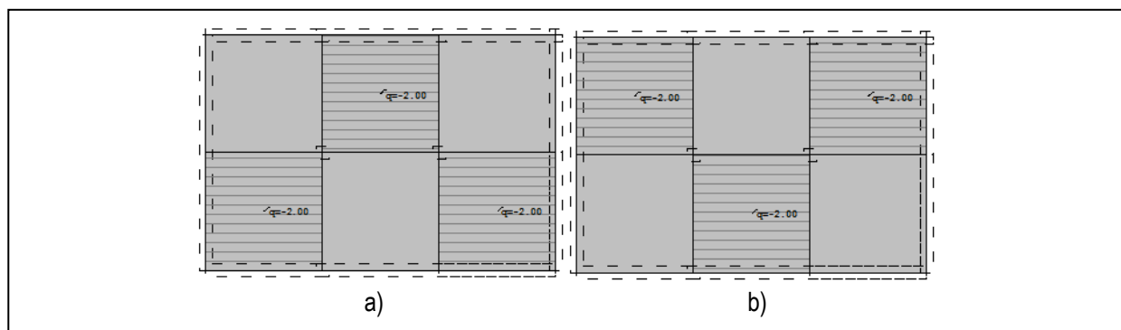
Slika 4 – Način modeliranja korisnog opterećenja na ploči 1 a) korisno opterećenje q_1 , b) korisno opterećenje q_2
