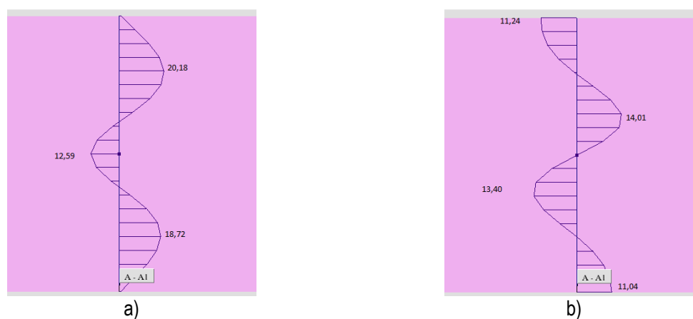
Slika 6 – Moment savijanja M_y u presjeku 1-1 (a) i poprečna sila V_{z,y} (b)
