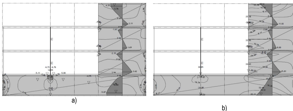
Slika 9 – Presjek 4-4 moment savijanja M x (a) i moment savijanja M y (b)
