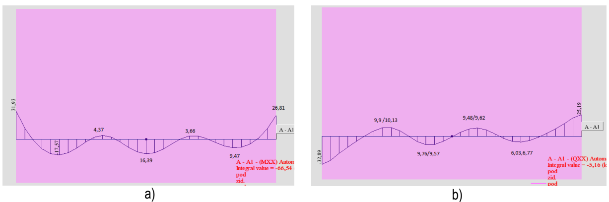
Slika 8 – Presjek 3-3 moment savijanja M_x (a) i poprečna sila V_{z,x} (b)
