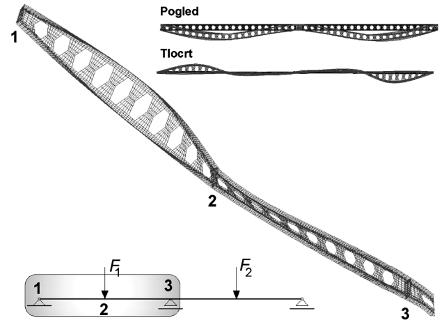
Slika 9. Prikaz deformacije modela u trenutku otkazivanja nosivosti Figure 9 The deformed model at the moment of reaching the ultimate load
