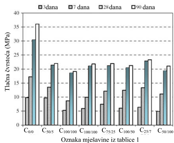
Slika 3. Tlačne čvrstoće betona [6]
