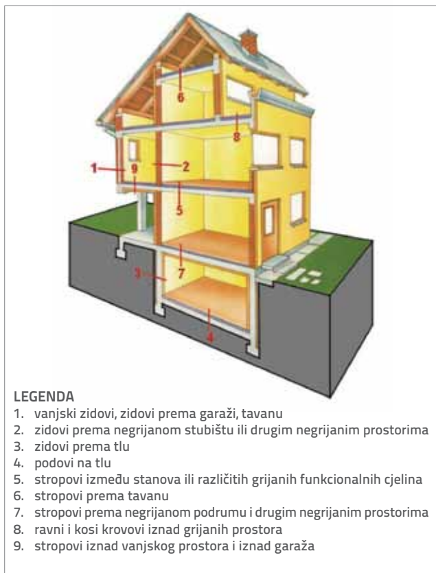
Slika 1. Omotač stambene zgrade
