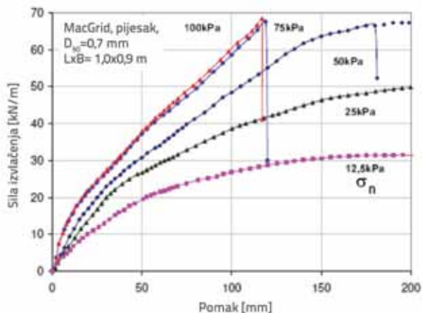
Slika 8. Porast sile izvlačenja pri povećanju normalnih naprezanja, [12]
