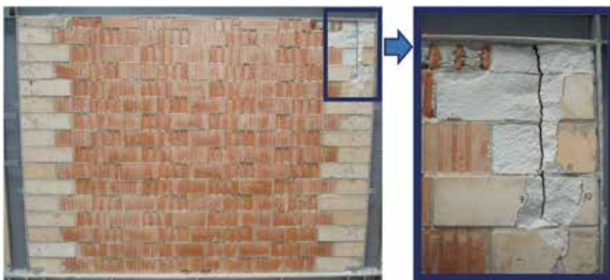
Slika 6. Fotografija uzorka CA-1 nakon sloma
