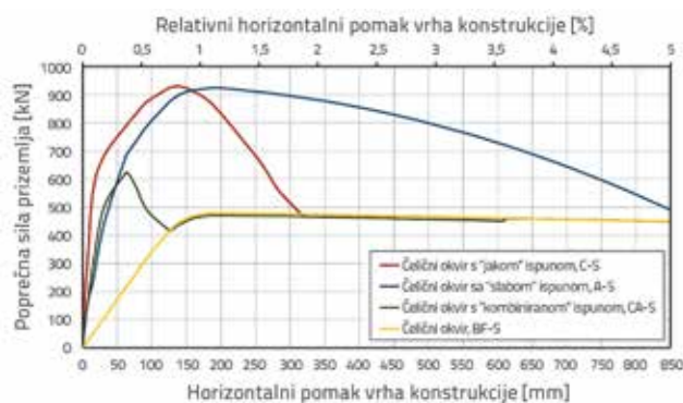
Slika 12. Dijagram poprečna sila prizemlja-horizontalni pomak vrha konstrukcije
