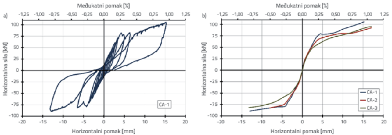
Slika 5. a) Histerezna petlja uzorka CA-1; b) Histerezne ovojnice uzorka CA- i
