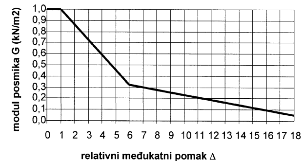
Slika 6. Idealizirani model nelinearnog ponašanja in-plane zida
