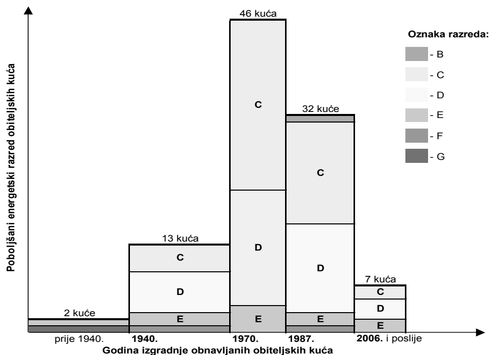
Slika 8. Poboļšani energetske razredi po godinama izgradnje kuća
