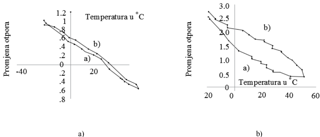
Slika 4.8 Promjena električne otpornosti: a) nakon prvog ciklusa smrzavanja i odmrzavanja pri temperaturama od -20 do 52^{\circ}\text{C} , te pri ponovnom hlađenju na -20^{\circ} i b) nakon zadnjega ciklusa smrzavanja i odmrzavanja pri temperaturama od -20 do 52^{\circ}\text{C} , te pri ponovnom hlađenju na -20^{\circ} [179]
