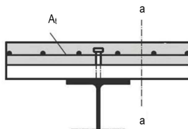
Slika 10.510 - Posmična površina a-a [5]
