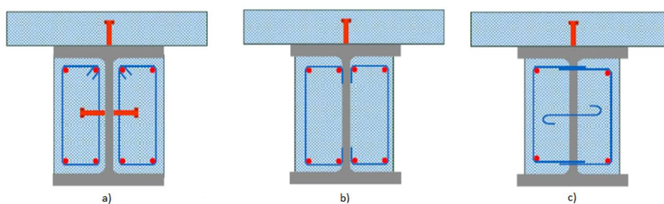
Slika 6.3 – Tipovi i razmještaj spona [7]
