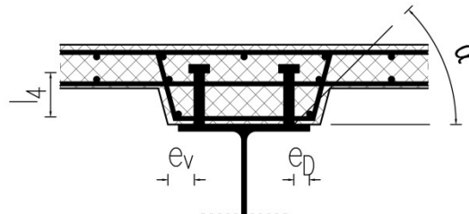
Slika 9.11 - Konstruktivske preporuke za betonsku vutu
