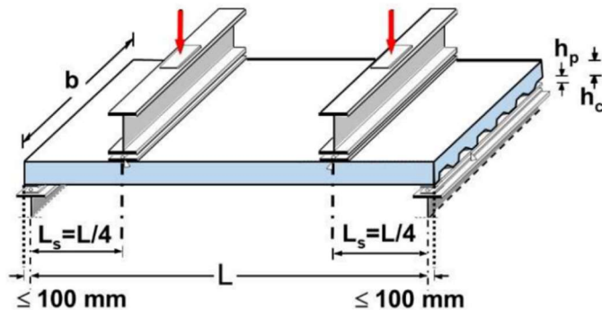
Slika 17.1 - Normirani postupak ispitivanja spregnute ploče [7]
