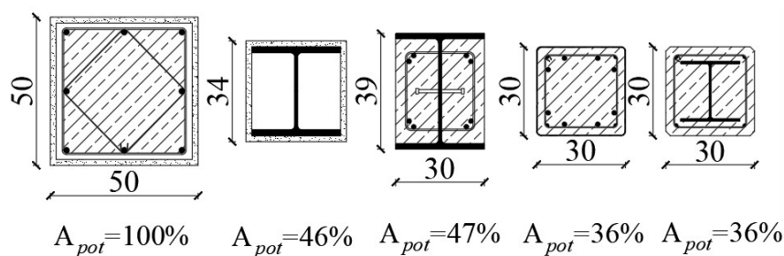
Slika 1.2 - Usporedba različito oblikovanih stupova unutar zgrade za jednake uvjete
