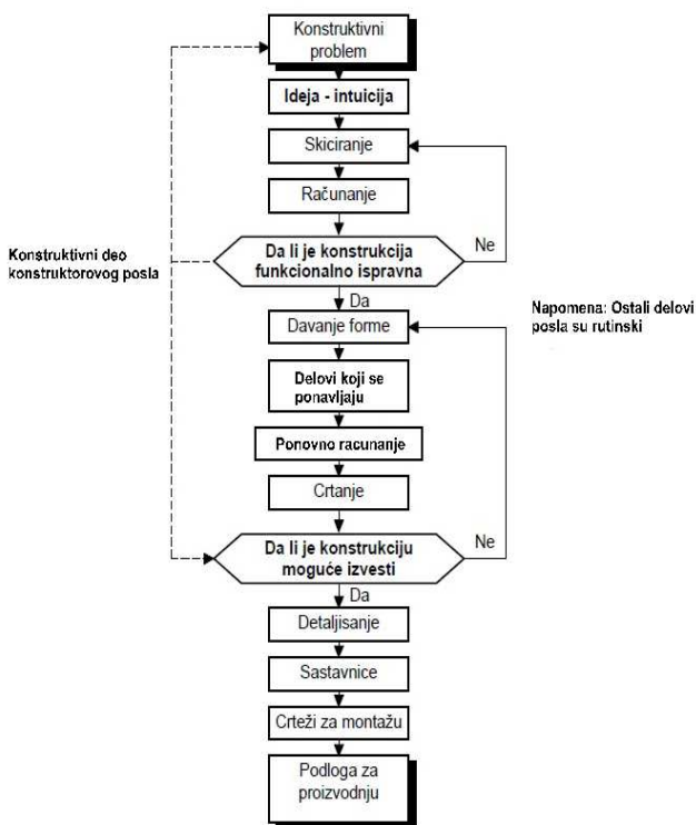
Slika 1. Šema procesa konstruisanja [2]
