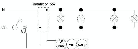
Slika 3. Mjerna točka snage rasvjete prostorije
