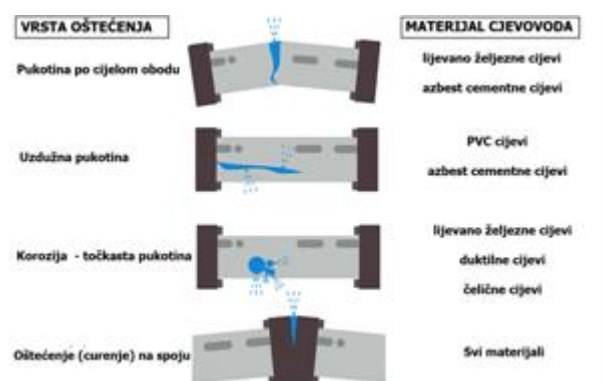
Slika 9. Vrste oštećenja prema materijalu cijevi [5]
