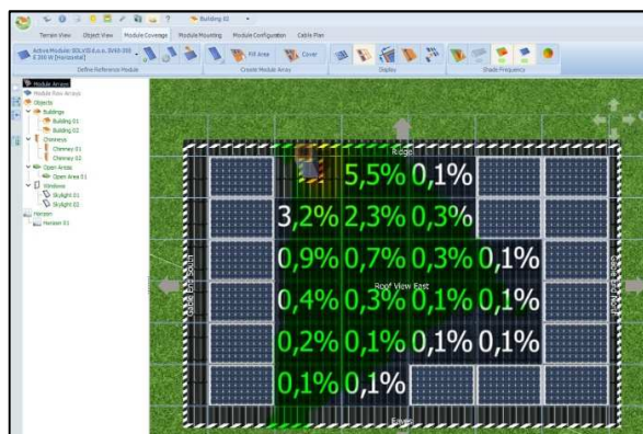
Slika 2. Zasjeenje dimnjakom
