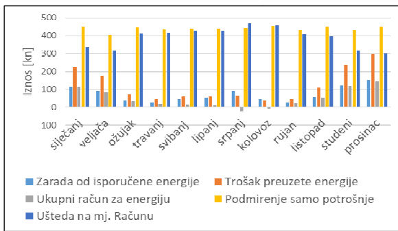
Slika 14. Novčani tokovi 4,5 kW i 2 sustava pohrane
