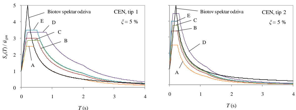
Slika 9. Spektri odziva definirani u europskim normama (CEN 2004a) i usporedba s Biotovim prijedlogom spektara odziva (prema Trifunac, 2006)
