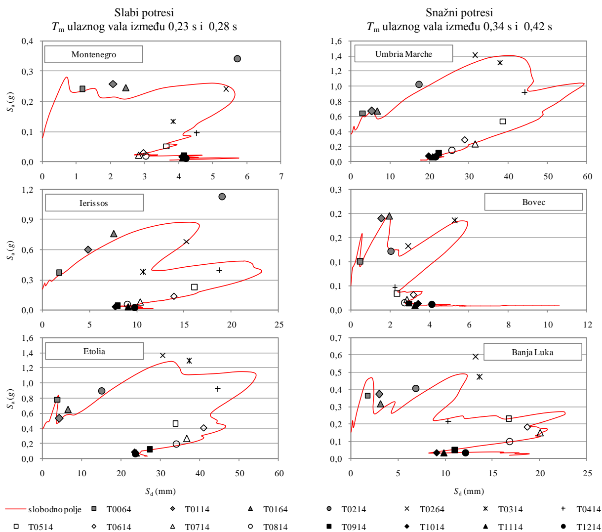
Slika 172. Usporedba potresnog odziva konstrukcija upetih u tlo 20RB-MS (crvena linija, konvencionalni spektar odziva) i plitko temeljenih pandana kojima je omogućeno klizanje i ljuljanje na tlu 20RB-MS (monokromatski markeri) pri djelovanju slabih i snažnih baznih ulaznih potresnih valova sa srednjim vrijednostima srednjih perioda
