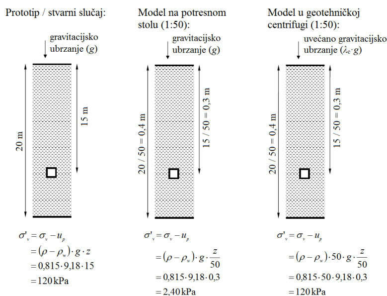
Slika 98. Usporedba modeliranja problema efektivnog napreznja prototipa u različitim uvjetima gravitacijskog ubrzanja (Knappett, 2013) (uredio autor)
