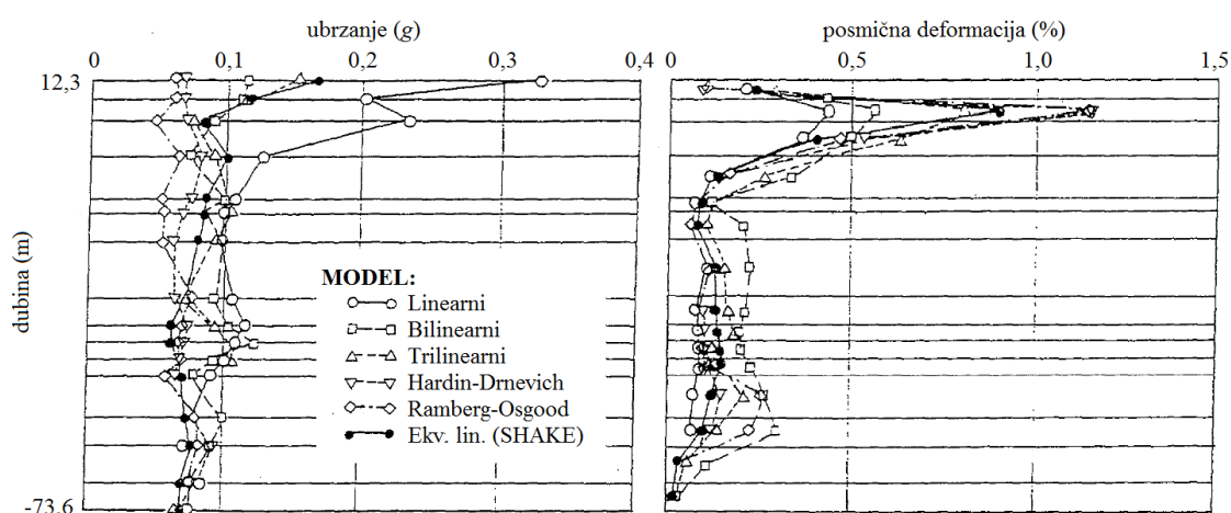
Slika 45. Usporedba procjene odziva tla primjenom različitih matematičkih modela za modeliranje tla (JSCE, 2000) (uredio autor)
