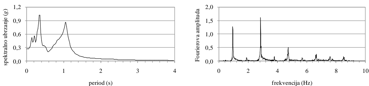
Slika 134. Spektar odziva ( lijevo ) i Fourierov spektar ( desno ) za obrađeni zapis T1F1E2
