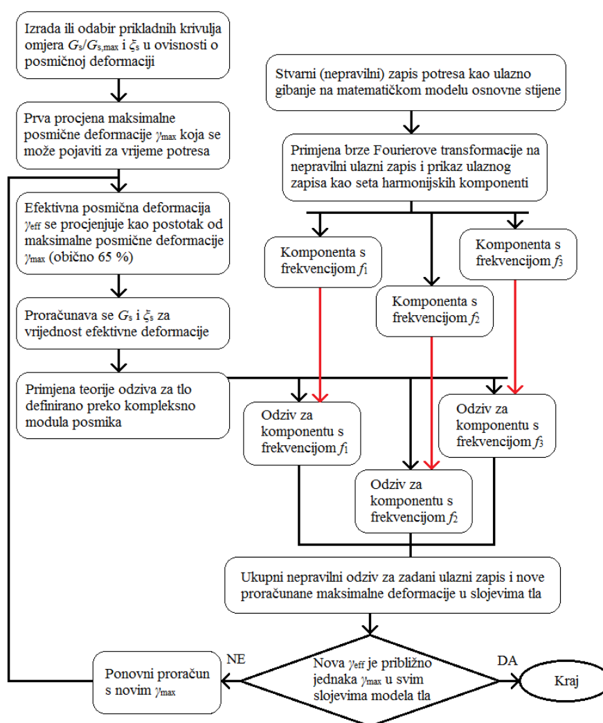
Slika 52. Tijek proračuna primjenom ekvivalentne linearne metode (prema Towhata, 2008)
