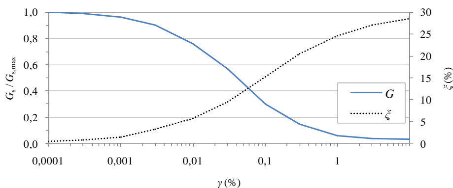
Slika 112. Srednja krivulja promjene omjera modula posmika i pripadajuća krivulja promjene prigušenja s obzirom na posmičnu deformaciju prema Seed, Wong, Idriss i Tokimatsu (1984)
