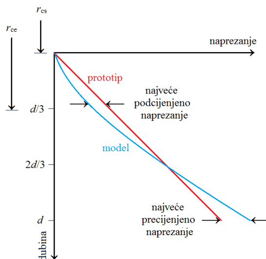
Slika 104. Usporedba promjene naprezanja po dubini modela tla u centrifugi i njemu odgovarajućeg prototipa (prema Taylor, 1995)
