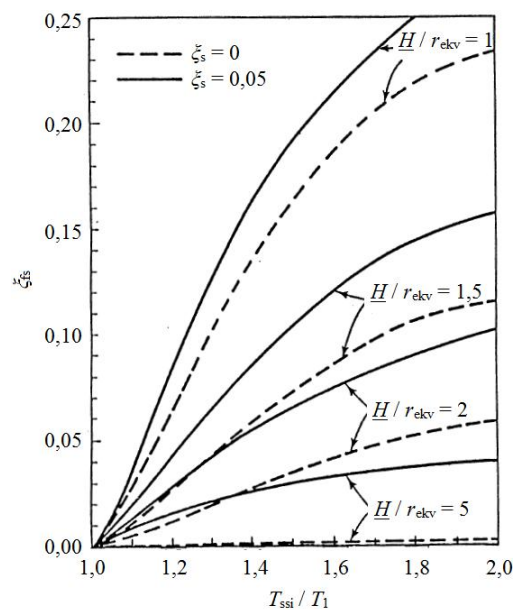
Slika 40. Dijagram ovisnosti produljenja osnovnog perioda osciliranja konstrukcije zbog popustljivosti temeljnog tla i koeficijenta relativnog prigušenja za temeljno tlo (Veletsos, 1978) (uredio autor)
