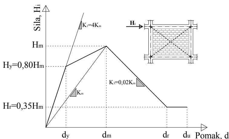
Slika 6.5 Krivulja odnosa sila-pomak prema modelu Decaninia (1993)
